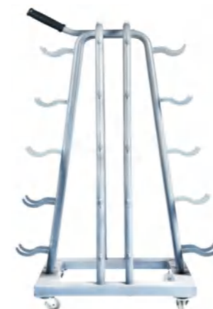
SC-80259 大手铃推车 Big size dumbbell go-cart Size:50°50°120cm QTY:1pc G.W.:20KGS MEAS:111°78°18CM 建议零售价：¥1200/pc
